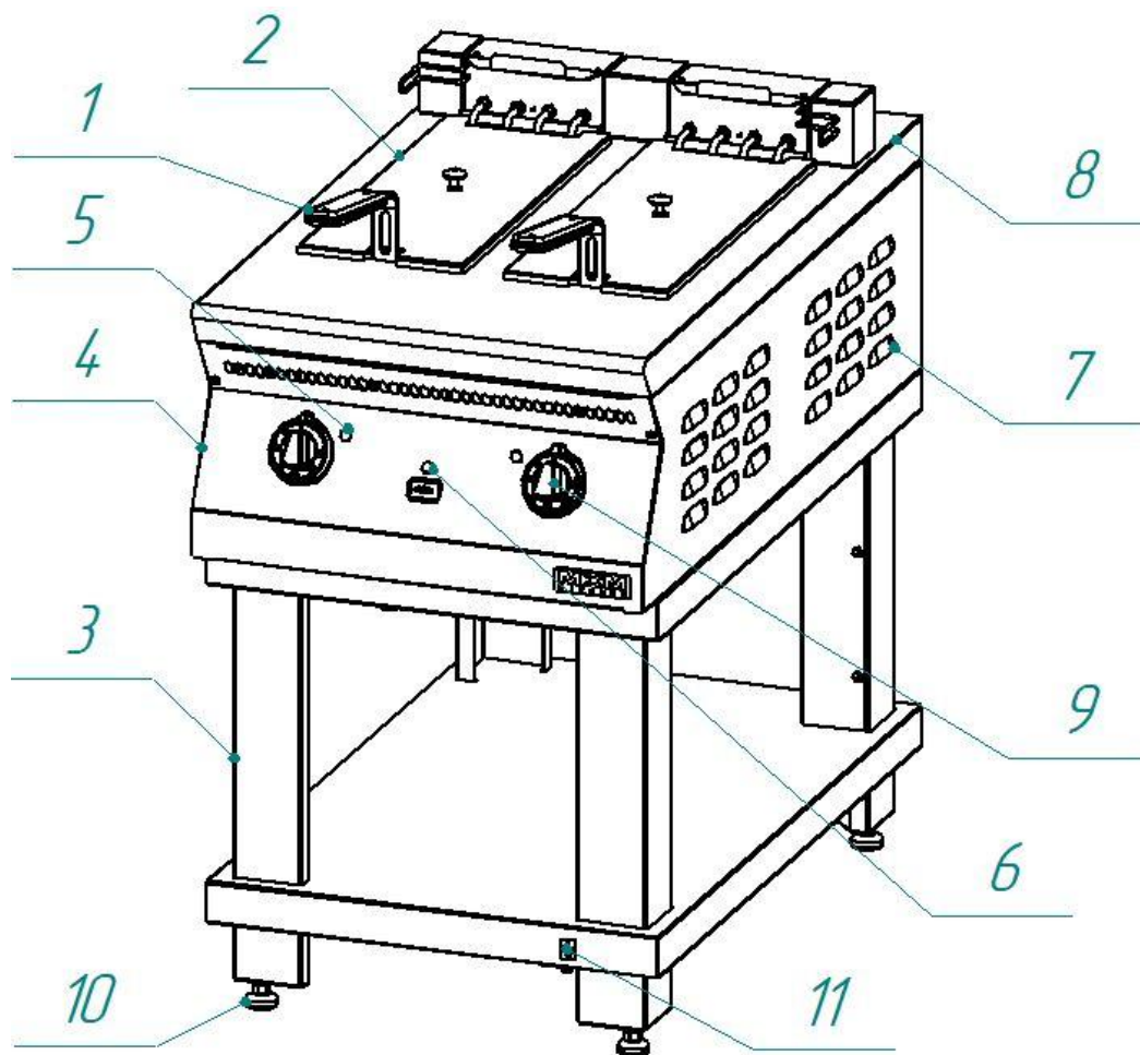
Рисунок 1 - Общий вид фритюра электрического ФЭК-90П
