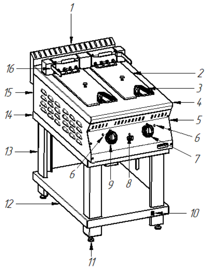
Рисунок 2 - Общий вид фритюрницы электрической кухонной ФЭК-90П-01
