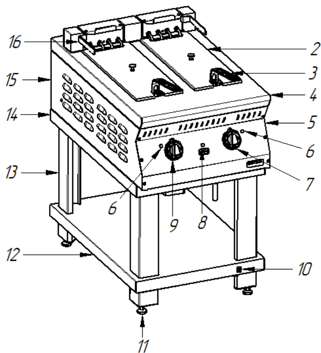
Рисунок 1 - Общий вид фритюрницы электрической кухонной ФЭК-90П
